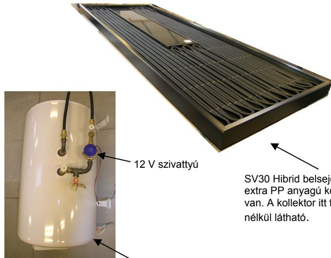
100 l hőtároló beépített hőcserélővel és idegenáramú anóddal
